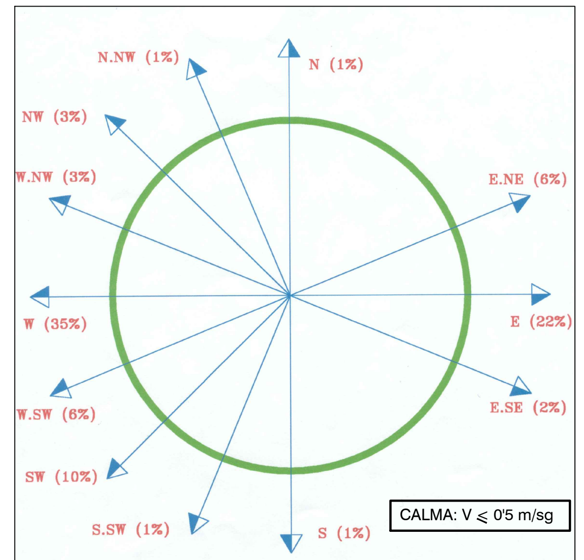
ROSA DE LOS VIENTOS FRECUENCIA DE LA DIRECCION DEL VIENTO EN TODO EL AÑO
